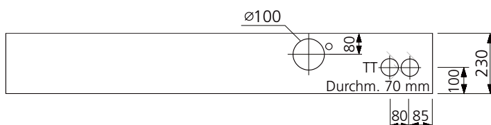
Schnitt A - A
