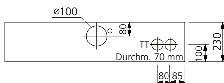
Schnitt A - A
